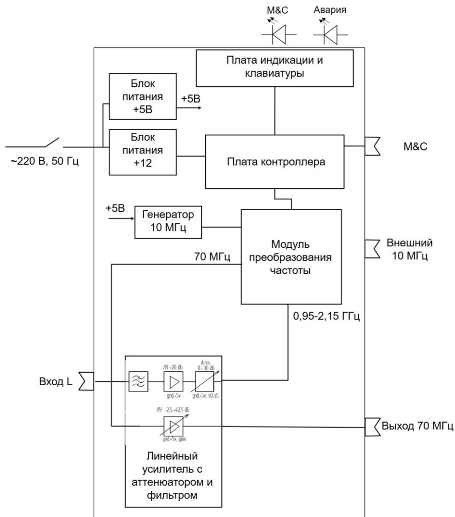
Рисунок 2 – Структурно-функциональная схема ПЧ «вниз»
